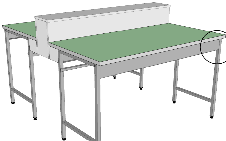
Détail : Fixation du bandeau métallique Plaque de fixation
